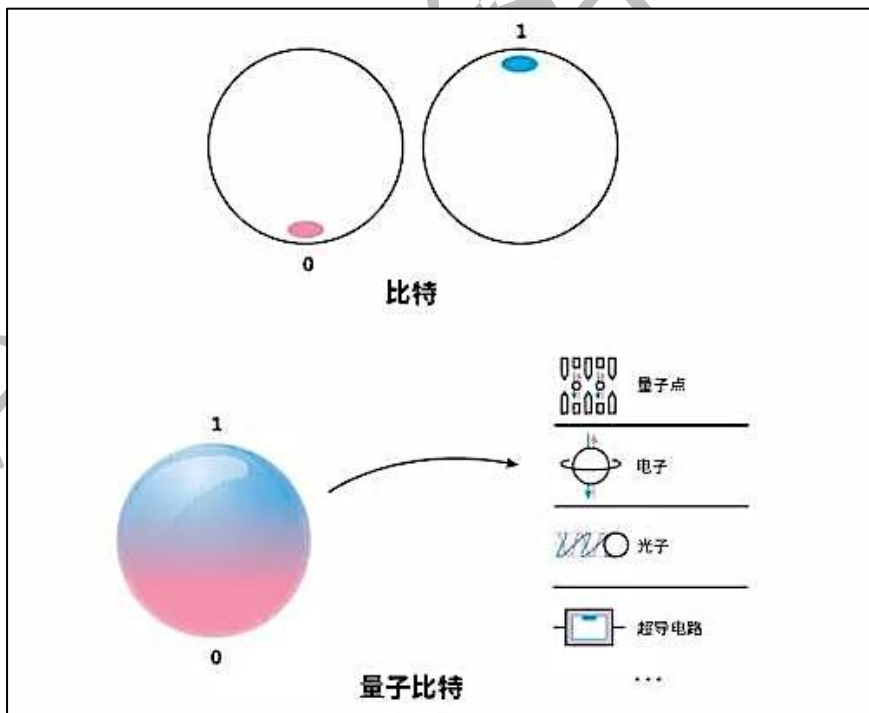
图 1 量子比特的概念示意图
