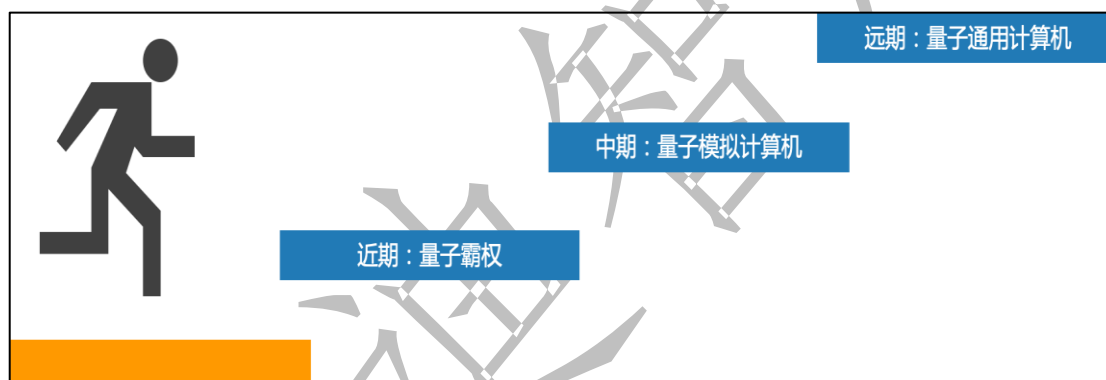
图 8 量子计算发展路线图
